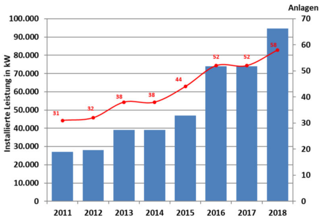
Abb. 2: Entwicklung der Windenergienutzung im Landkreis Göttingen
