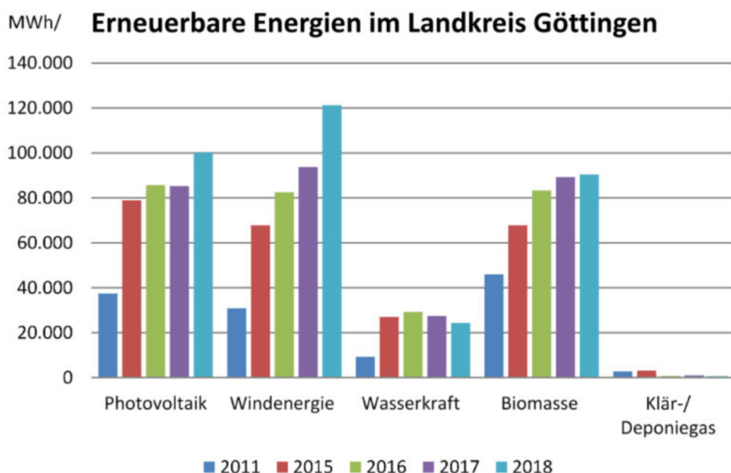
Abb. 1: Entwicklung der erneuerbaren Energien im Landkreis Göttingen
