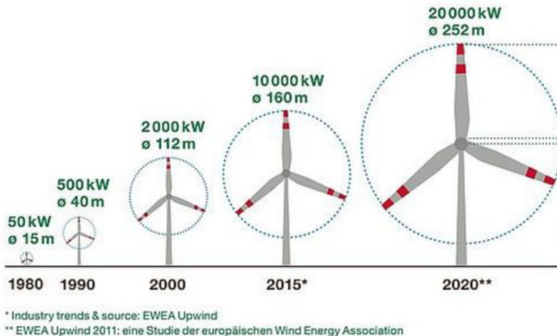
Abb. 4: Größenentwicklung von Windenergieanlagen (verändert, https://www.energie-experten.org/erneuerbare-energien/windenergie.html )
